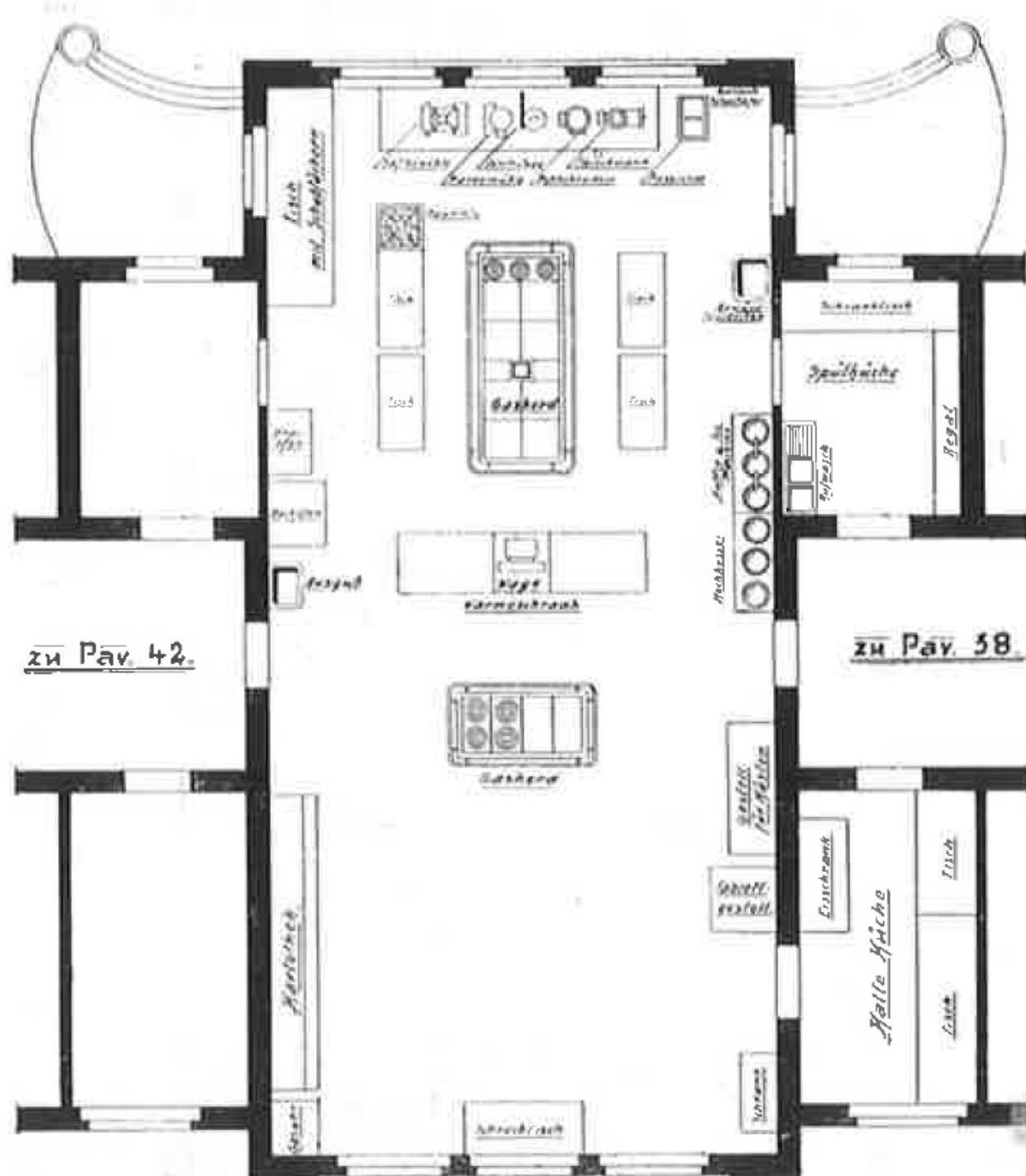
Grundriß der Diätküche
